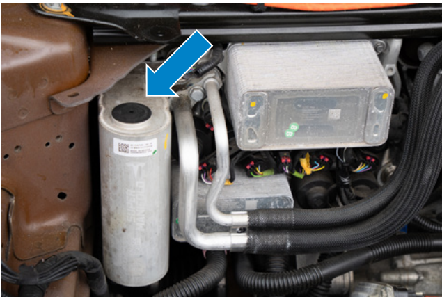
Einbausituation im Supermanifold im Model 3
